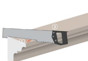
2_SEČENJE FASADNE LAJSNE
