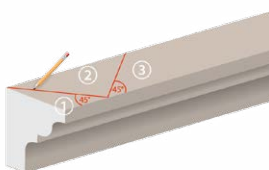
1_OBELEŽAVANJE LINIJA SEČENJA
